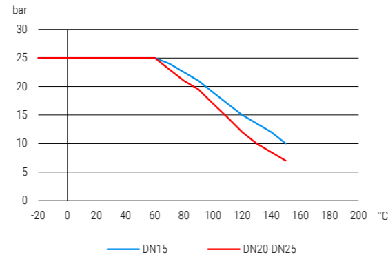
Druck-Temperatur-Diagramm pressure-temperature-diagram
